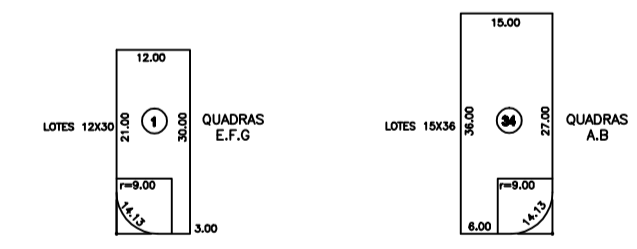
CONCORDÂNCIA DOS VERTICES DAS QUADRAS ESCALA 1:175
