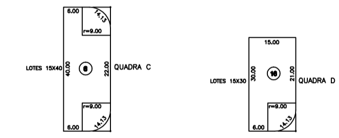
CONCORDÂNCIA DOS VERTICES DAS QUADRAS ESCALA 1:175
