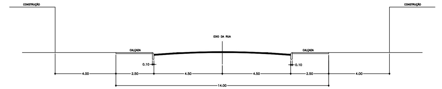
SESSÕES TRANSVERSAIS DAS VIAS ESCALA 1:175
