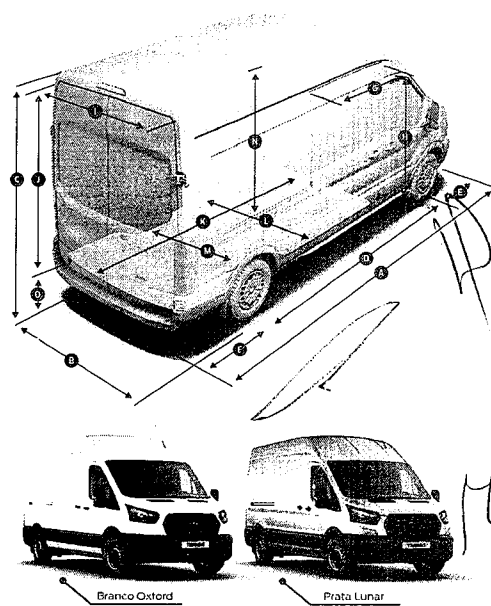
L2H3 Furgão com capacidade volumétrica de carga de 10,7m³ e categoria "B" de habilitação.
