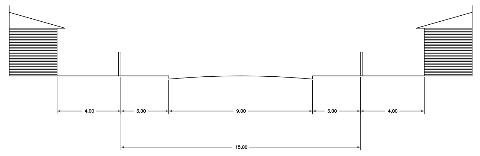
PERFIL TRANSVERSAL-VIAS DE 15,00m ESCALA 1:100
