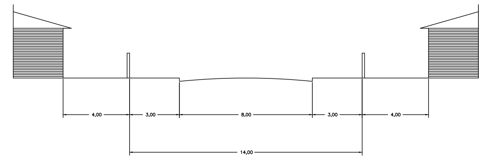
PERFIL TRANSVERSAL-VIAS DE 14,00m ESCALA 1:100
