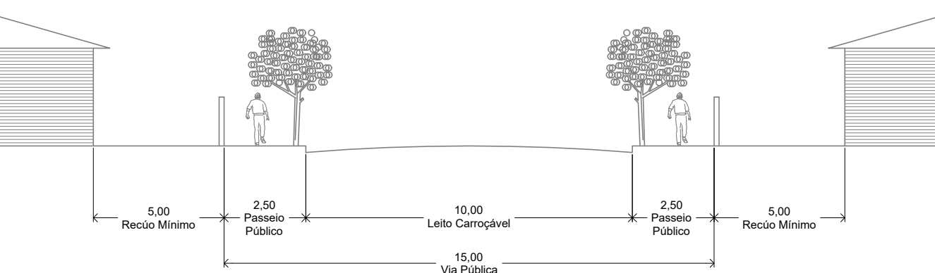
PERFIL TRANSVERSAL DAS VIAS SEM ESCALA
